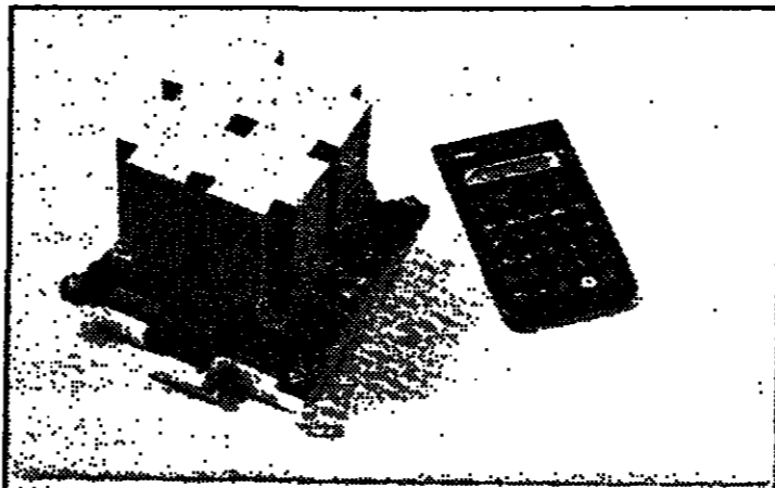
Le cœur des nouveaux ordinateurs IBM. L'unité centrale tient sur un support en aluminium portant 118 circuits intégrés. Un radiateur la surmonte qui évacue la chaleur dissipée par ces circuits. La calculatrice donne l'échelle.
